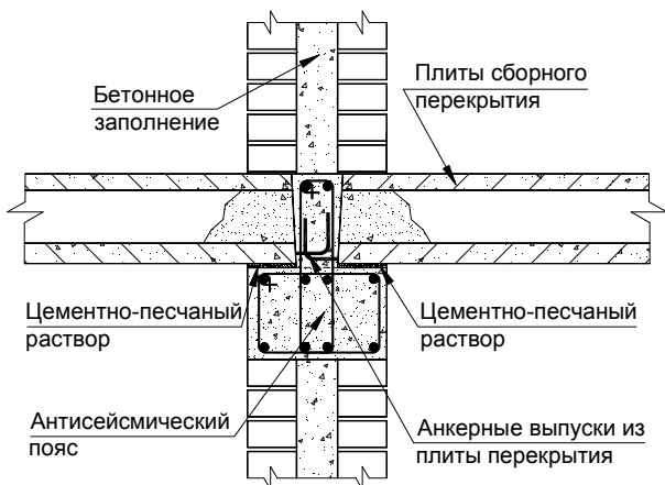
Рисунок 4.5 – Примеры устройства железобетонных антивсейсмических поясов в уровнях междуэтажных сборных перекрытий
