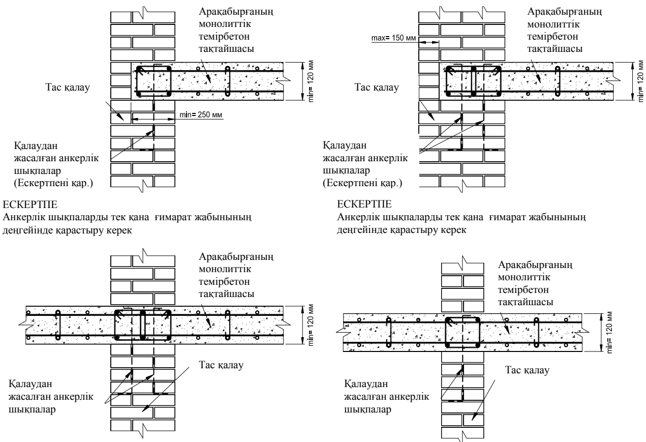
4.9-сурет – Арақабырғаның монолиттік темірбетон тақтайшаларын тас қабырғалармен қосудың мысалдары
