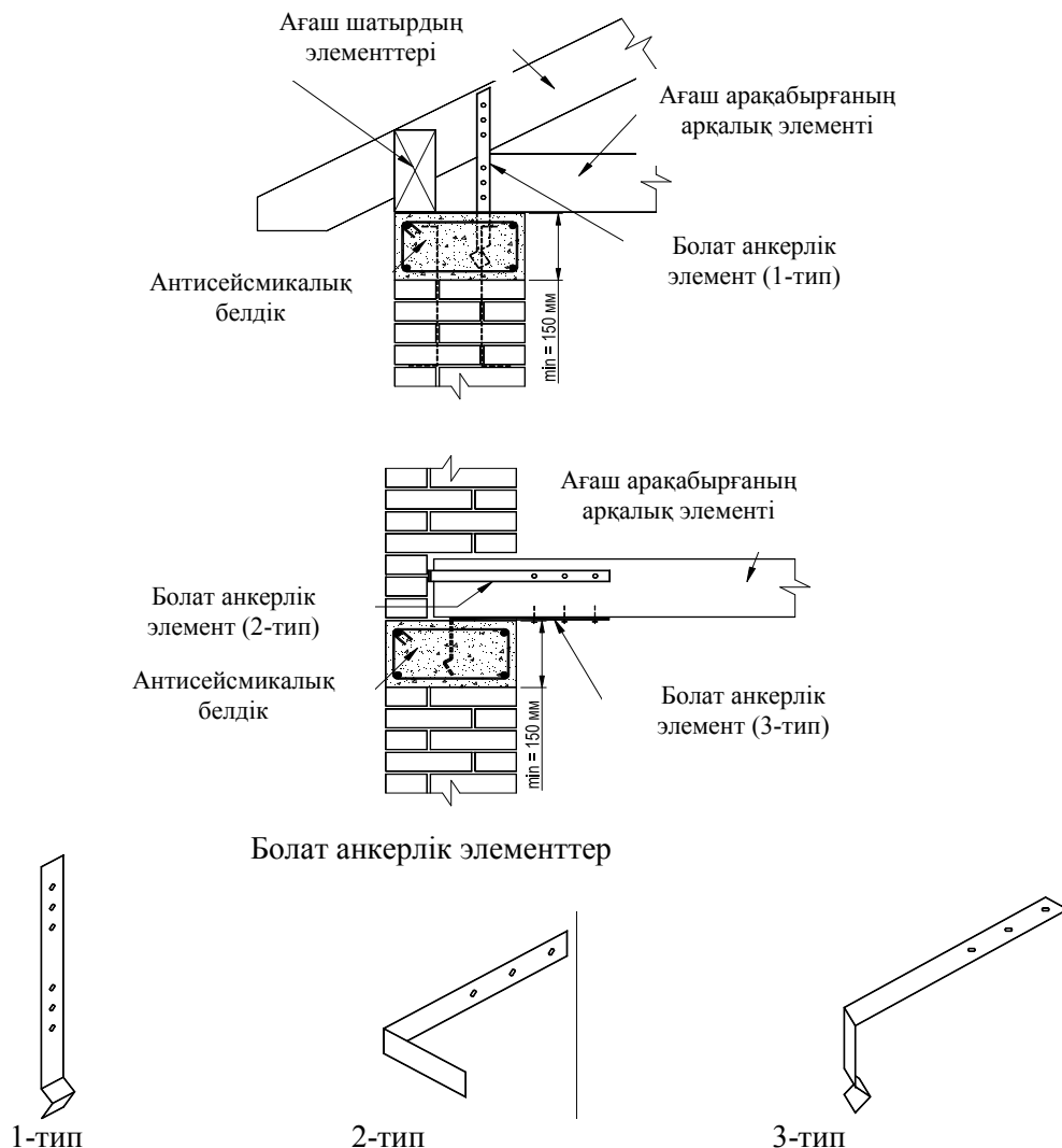
4.1-сурет – Ағаш арақабырғалардың арқалық элементтерін бекіту тораптарының мысалдары
