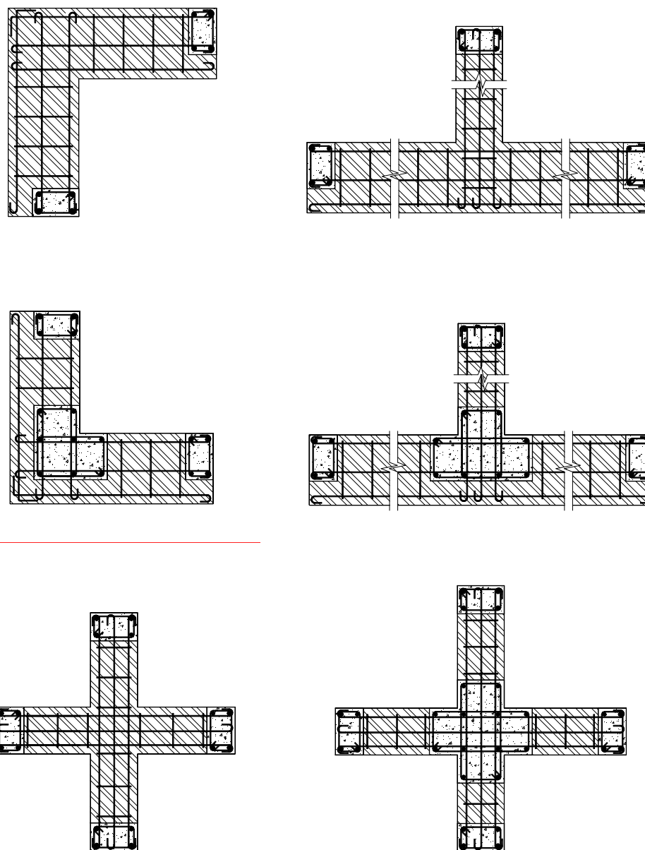
Рисунок 3.7 – Фрагменты каменной кладки стен с ограничивающими вертикальными элементами
