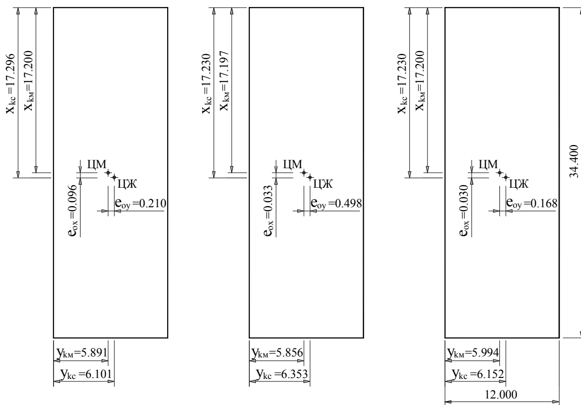
А3-сурет – Қабатаралық арақабырғалар деңгейіндегі массалар мен қаттылық орталықтарының күйі
