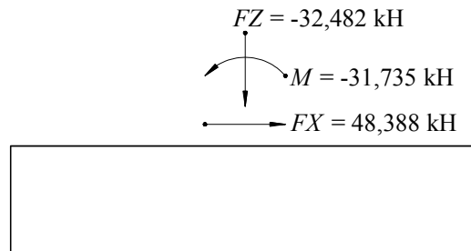
Рисунок А.9 – Схема нагрузок, действующих на рассматриваемый простенок в его плоскости при комбинации нагружения №29
