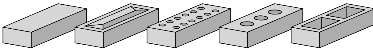
Рисунок 2.2– Характерные геометрические формы элементов каменной кладки (полнотелый, полнотелый с выемкой, перфорированный, пустотелый)
