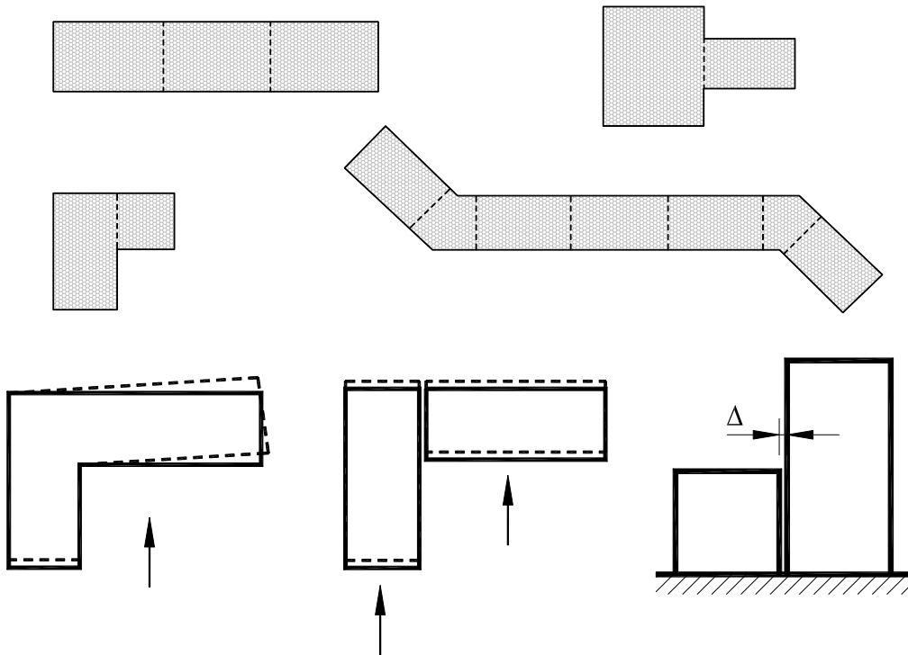
Рисунок 6.1 – Схемы расположения антисейсмических швов
