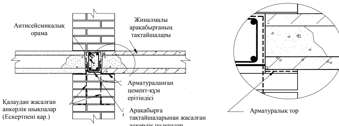
4.4-сурет – Темірбетон антисейсмикалық орамалардың қабатаралық жиналмалы арақабырғалардың деңгейінде орналасуының мысалдары
