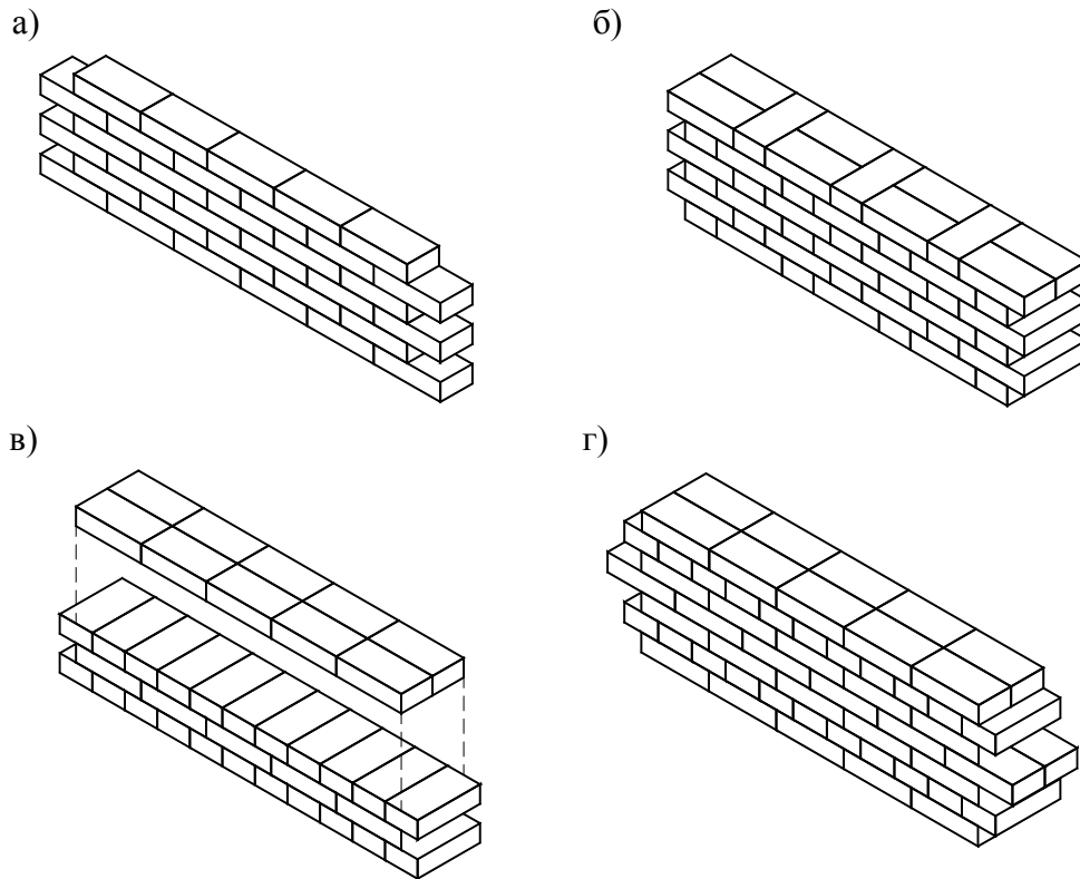
Рисунок 2.3 – Примеры некоторых цепных (а, б, в) и трехрядных (г) систем перевязки в каменных кладках из полнотелого глиняного кирпича
