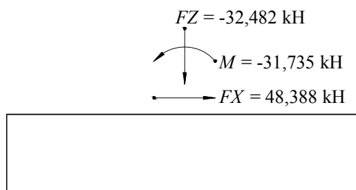
А.9-суреті – № 29 жүктеу комбинациясы кезінде оның жазықтығындағы қарастырылып отырған аралық қабырғаға әрекеттенетін жүктемелердің схемасы
