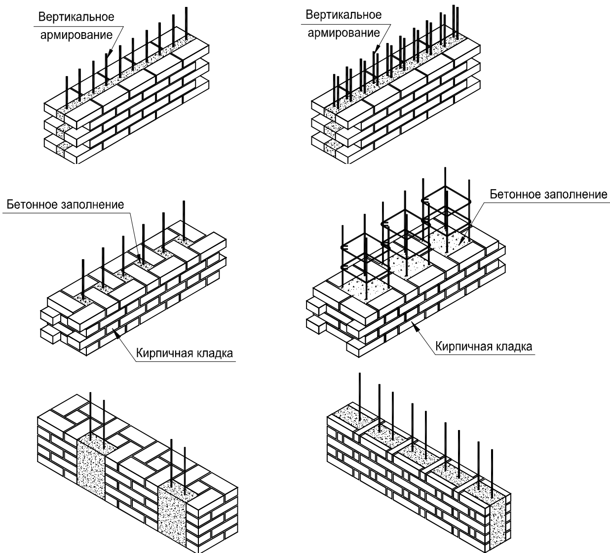
Рисунок 3.9 – Фрагменты стеновых конструкций из армированной каменной кладки, выполняемой с применением пустотелых элементов
