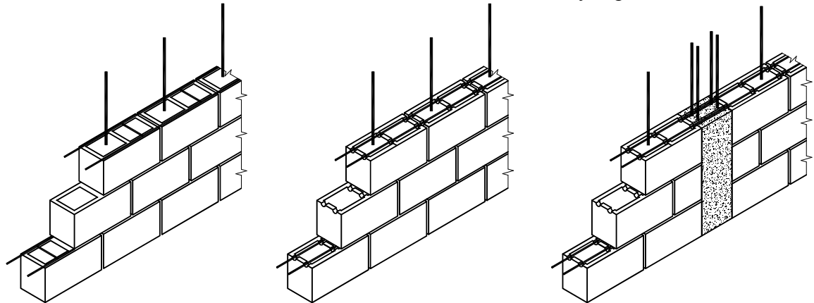
3.9-сурет – Бос денелі элементтерді қолдану арқылы орындалған арматуралық тас қалаулардан жасалған қабырғалық конструкциялардың фрагменттері
