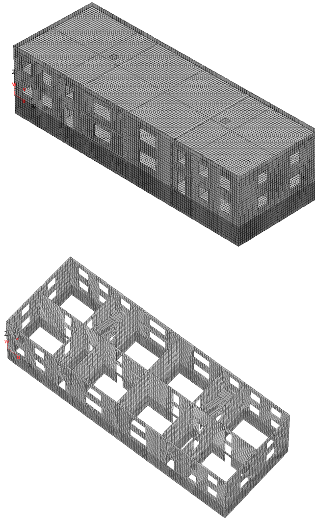
А2-сурет – Ғимараттың соңғы-элементтік есептік моделі
