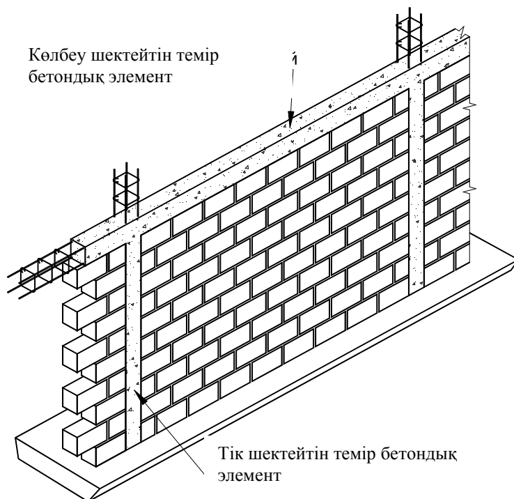
3.3-сурет – Шектейтін тас қалаудан жасалған қабырғалық конструкцияның қағидаттық конструктивтік шешімі
