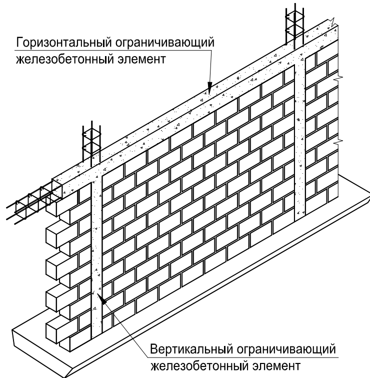
Рисунок 3.3 – Принципиальное конструктивное решение стеновой конструкции из ограничиваемой каменной кладки
