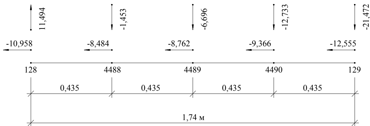
Рисунок А.7 – Результирующие величины сил в узлах конечных элементов при комбинации нагружения №30
