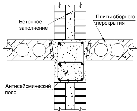
Рисунок 4.5 – Примеры устройства железобетонных антивсейсмических поясов в уровнях междуэтажных сборных перекрытий
