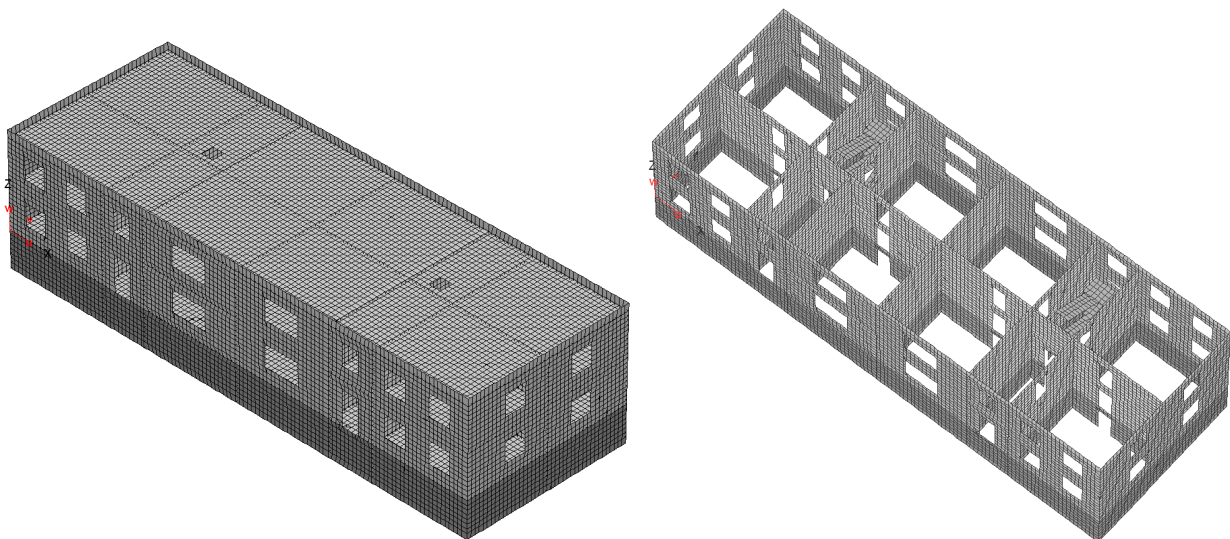
Рисунок А.2 – Конечно-элементная расчетная модель здания
