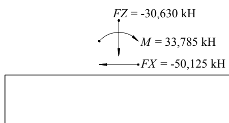
А.8-суреті – № 30 жүктеу комбинациясы кезінде оның жазықтығындағы қарастырылып отырған аралық қабырғаға әрекеттенетін жүктемелердің схемасы
