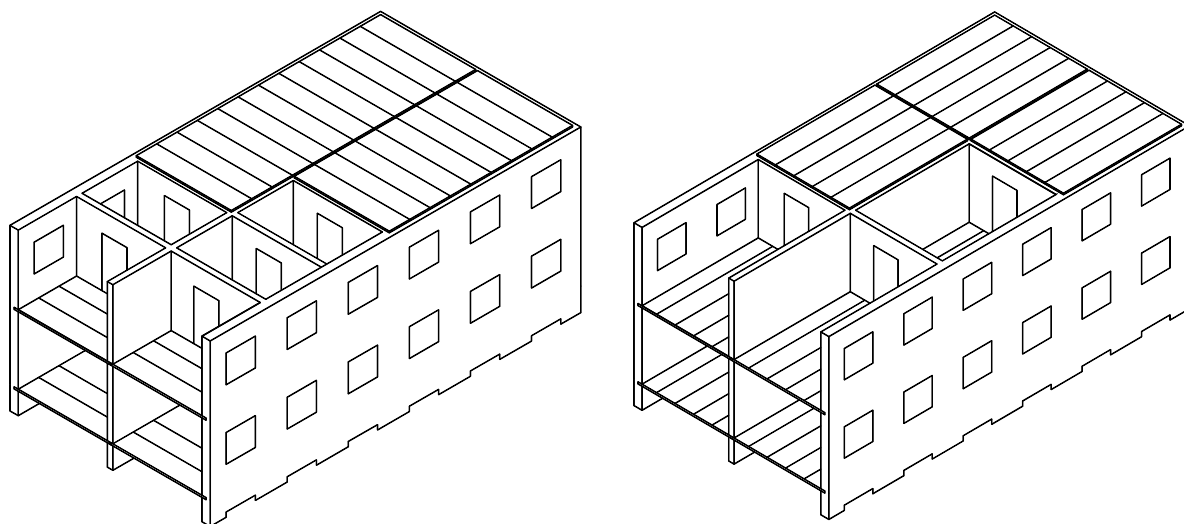
2.1-сурет – Бойлық (а)) және көлденең (б)) қабырғалардағы жиналмалы темірбетондық арақабырға тақтайшаларына тірелген айқасқан-қабырғалы конструктивтік жүйелер
