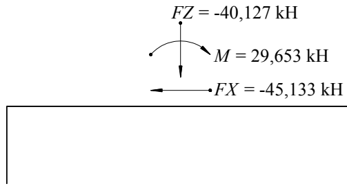
А.10-суреті – № 7 жүктеу комбинациясы кезінде оның жазықтығындағы қарастырылып отырған аралық қабырғаға әрекеттенетін жүктемелердің схемасы
