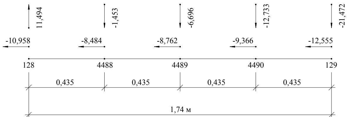
А.7-суреті – № 30 жүктеу комбинациясы кезінде соңғы элементтер тораптарындағы қорытындылайтын шамалар
