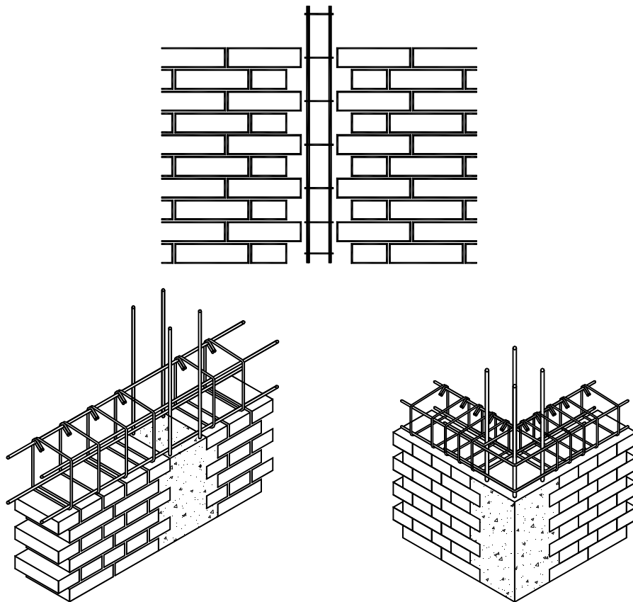
Рисунок 3.3 – Принципиальное конструктивное решение стеновой конструкции из ограничиваемой каменной кладки
