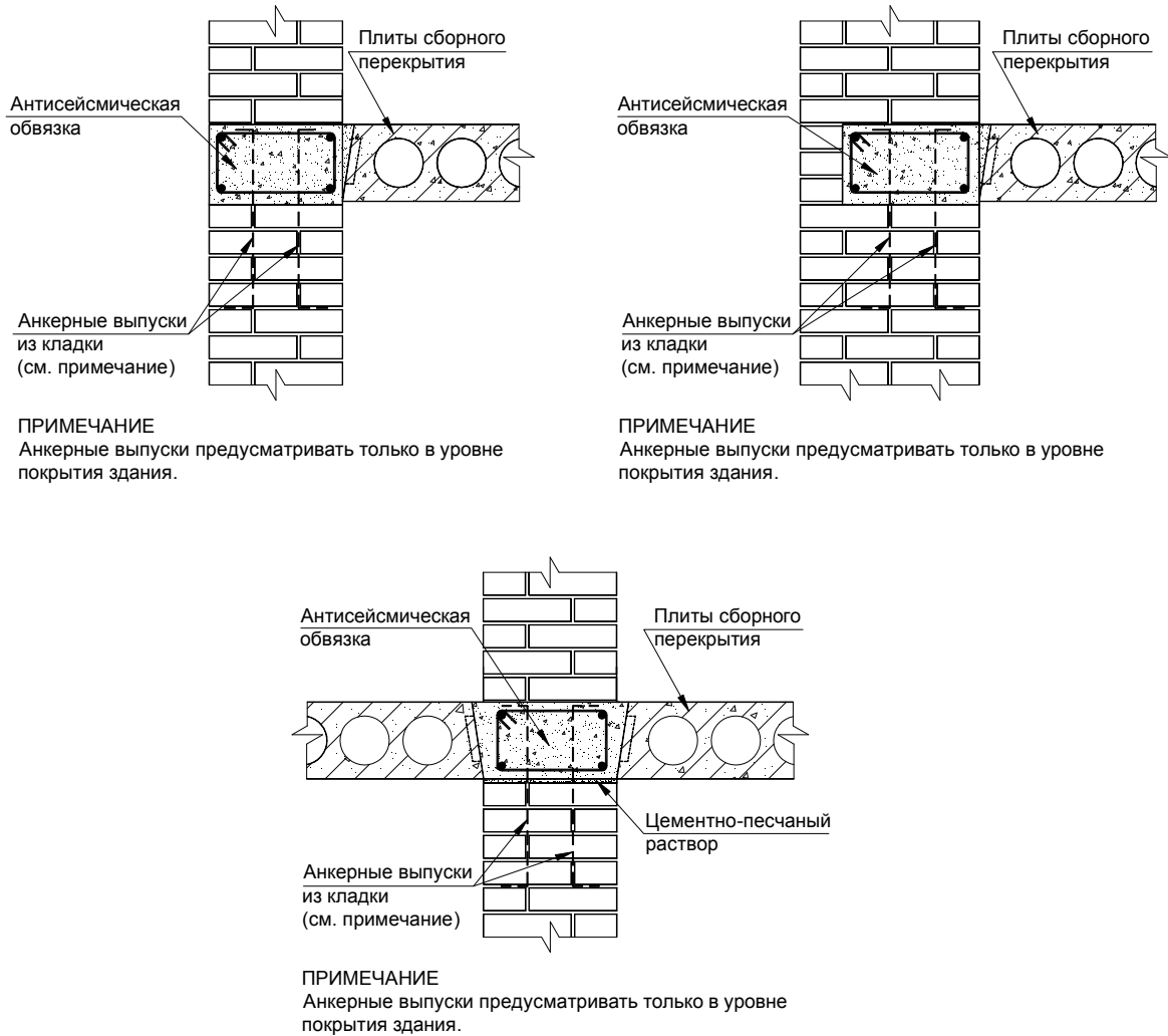
Рисунок 4.4 – Примеры устройства железобетонных антисейсмических обвязок в уровнях междуэтажных сборных перекрытий (продолжение)
