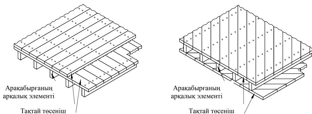
4.2-сурет – Арқалық бойынша қос тақтай төсеніш
