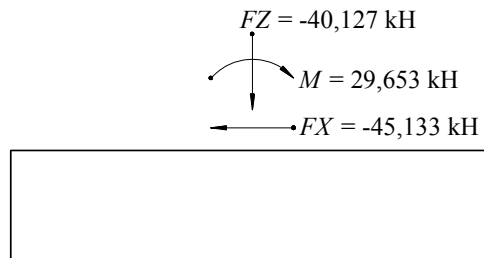
А.11-суреті – № 4 жүктеу комбинациясы кезінде оның жазықтығындағы қарастырылып отырған аралық қабырғаға әрекеттенетін жүктемелердің схемасы
