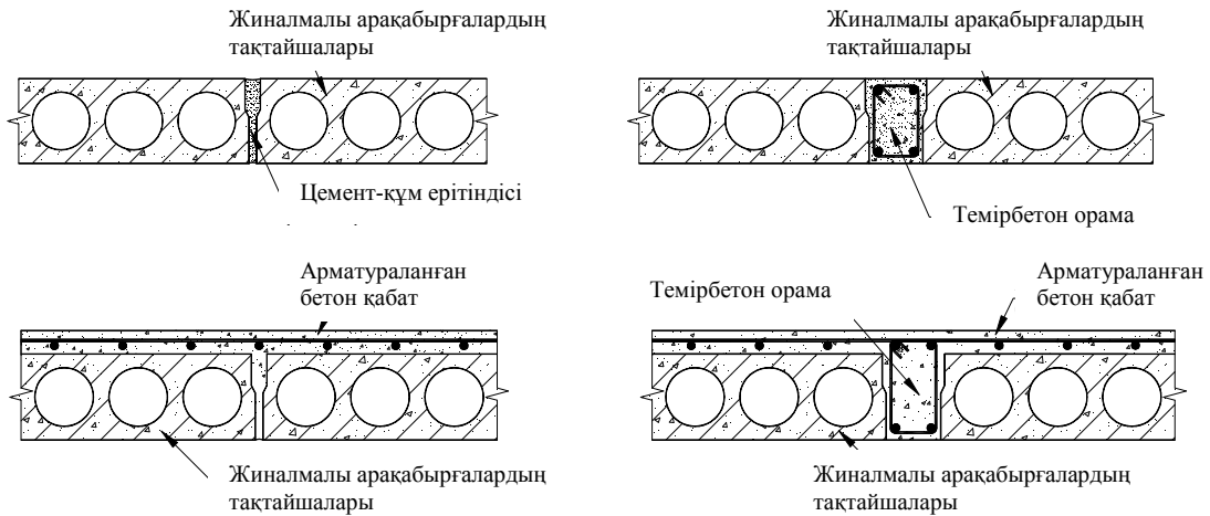
4.6-сурет – Жиналмалы темірбетон арақабырғалардың немесе жабындардың қаттылығын ұлғайтатын конструктивтік шаралардың мысалдары
