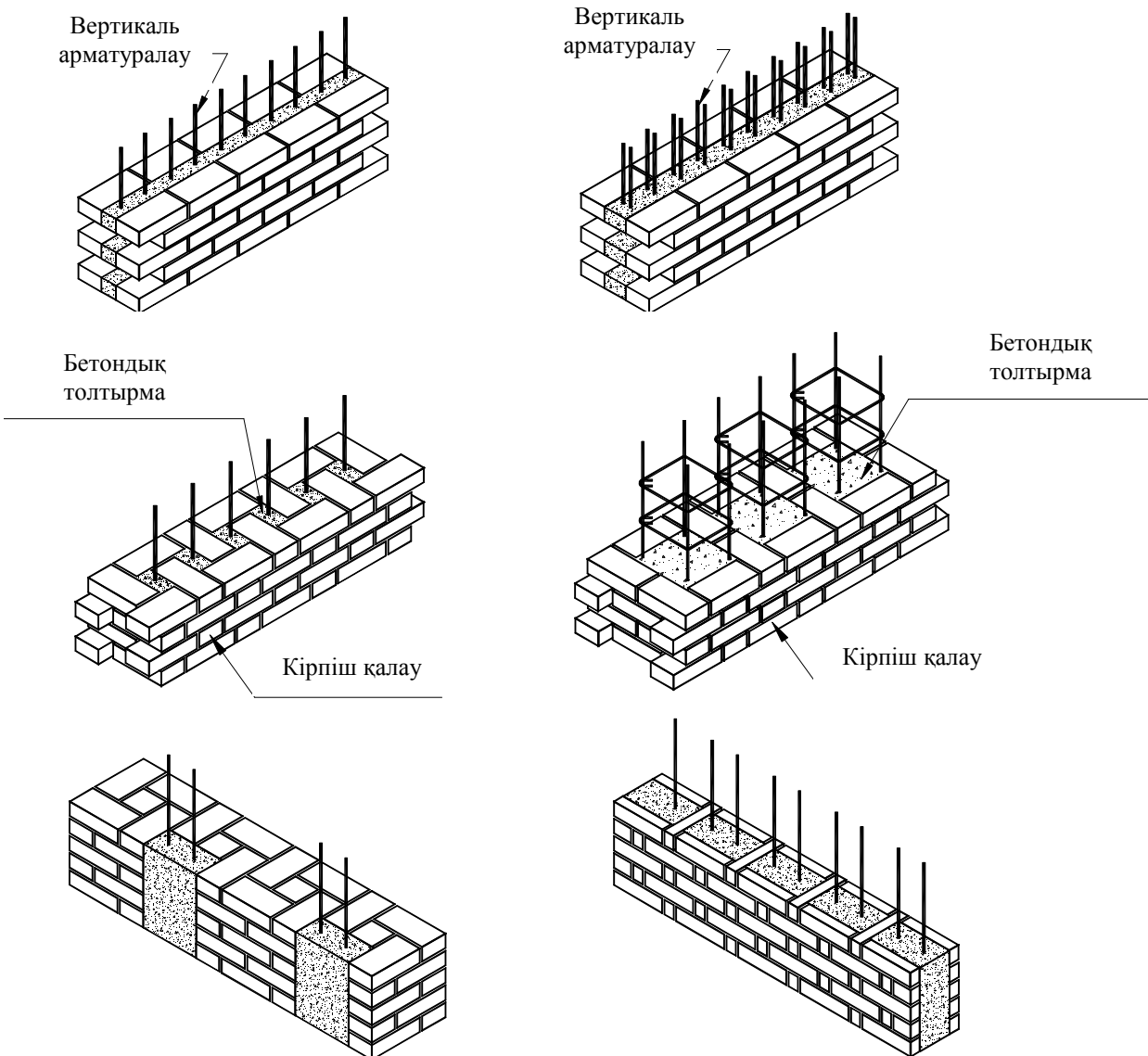
3.10-сурет – Толық денелі элементтерді қолдануы бар арматуралық тас қалаулардың конструктивтік шешімдерінің нұсқалары
