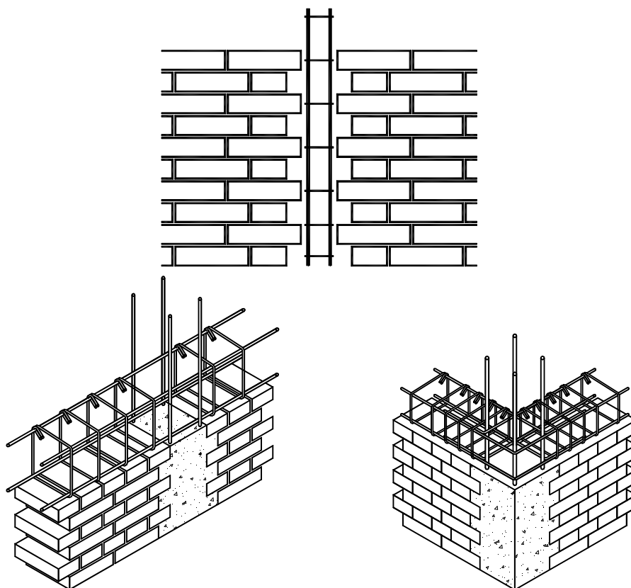
3.4-сурет – Вертикаль шектейтін элемент пен қалаудың арасындағы байланысты қамтамасыз ететін конструктивтік шешімнің мысалы
