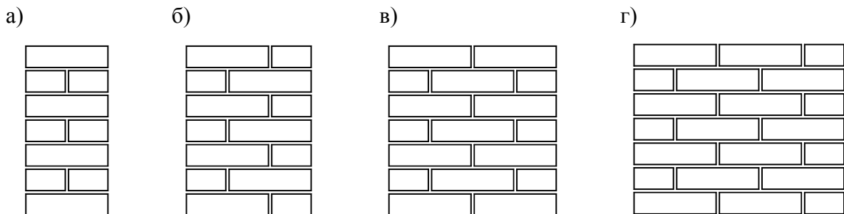
Сурет 2.3 – Бір қабатты қабырғаның тас қалауының қалыңдығы: а) 1 элементке; б) 1\frac{1}{2} элементке; в) 2 элементке; г) 2\frac{1}{2} элементке
