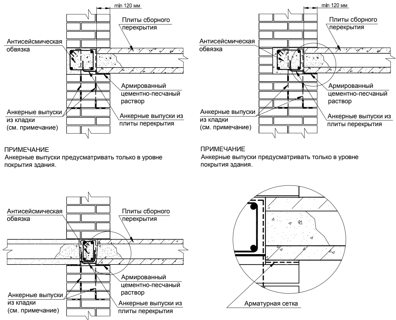
Рисунок 4.4 – Примеры устройства железобетонных антисейсмических обвязок в уровнях междуэтажных сборных перекрытий
